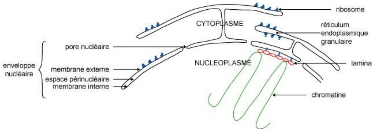
Figure 3-2 Enveloppe nucléaire
